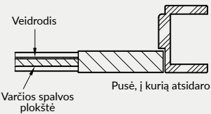
Estra 10 durys „reverso“ variante
