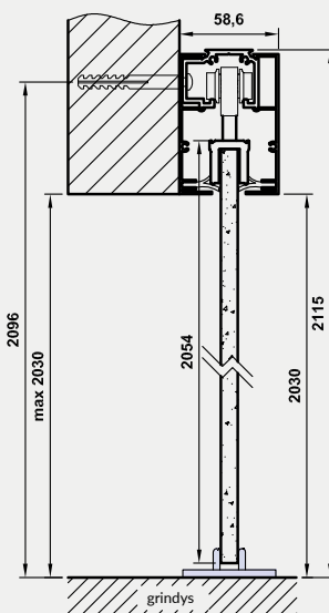
A – vertikalus „Spazio TP“ sistemos vertikalus pjūvis
