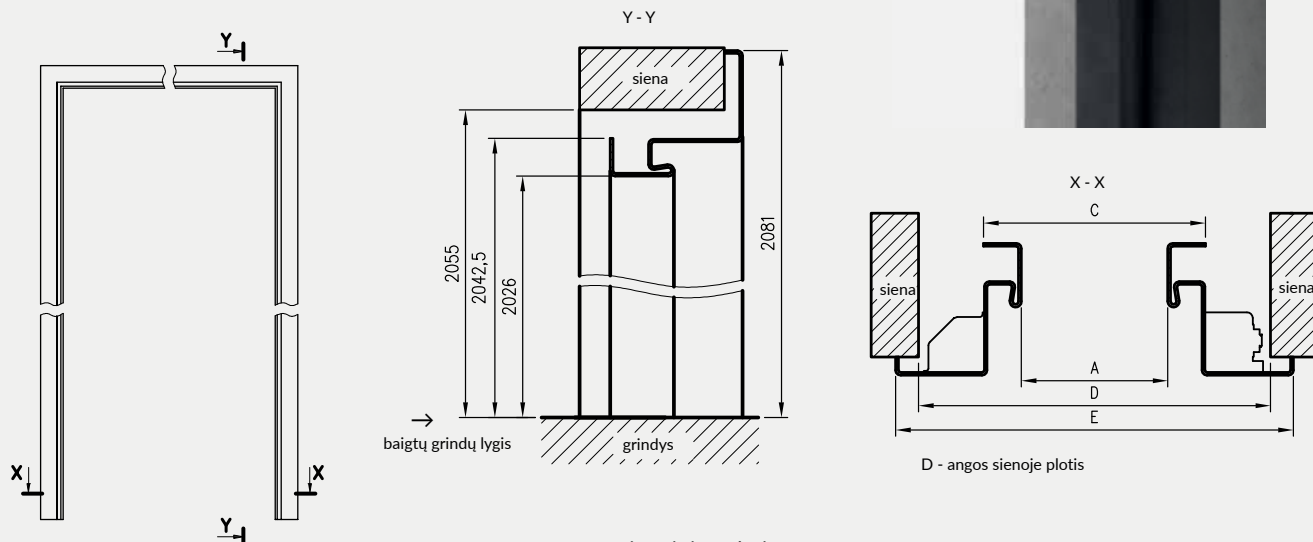
matmenys vienvėrėms durims
