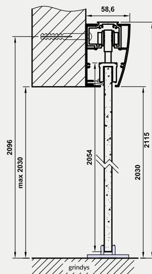
A – vertikalus „Spazio TO“ sistemos vertikalus pjūvis
