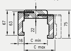
TUN su kamp. T63 pjūvis
