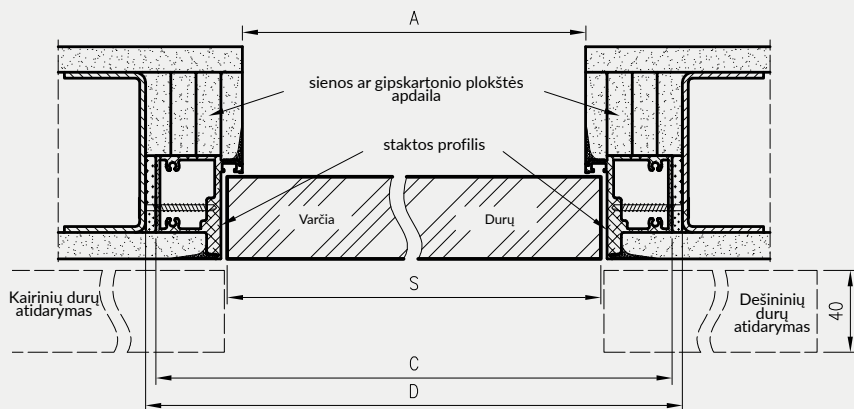
Sara Eco 2 lygiabriaunių durų – atsidarančių į išorę, skerspjūvis
