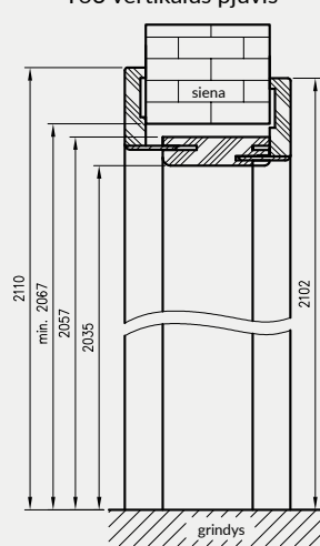
Reguliuojamo tunelio su kamp. T63 vertikalus pjūvis
