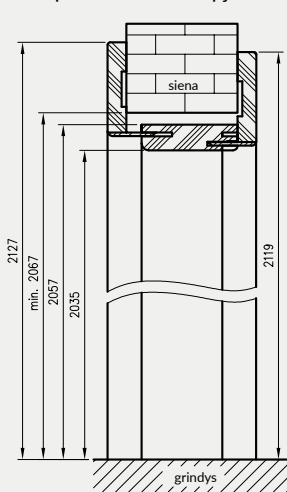
Reguliuojamo tunelio su kamp. T80 vertikalus pjūvis
