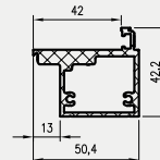
DRE profilis į išorę atsidarančioms lygiabriaunėms durims
