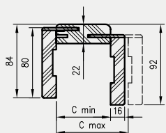
TUN su kamp. T63 pjūvis
