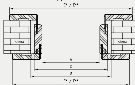
TUN skerspjūvis
