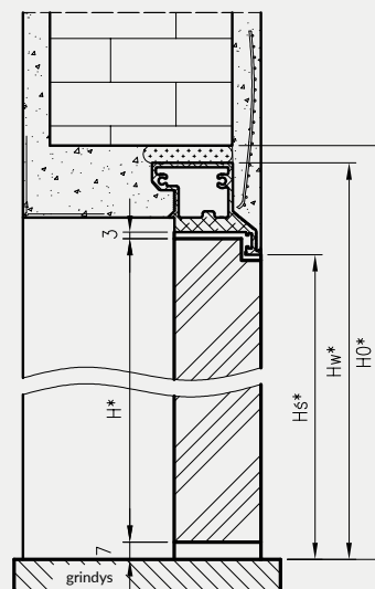
DRE profilis į vidų atsidarančioms durims su apversta užlaida
