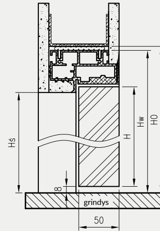
Vertikalus 50 mm lygiabriaunių durų vertikalus pjūvis – atsidarančios į išorę
