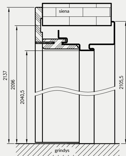
Y - Y Vertikalus pjūvis OSHB
