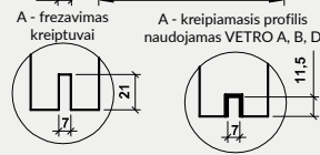
„Olimp EI60“ varčios**
