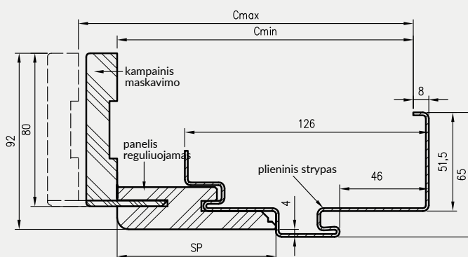
OSHB staktos profilis
