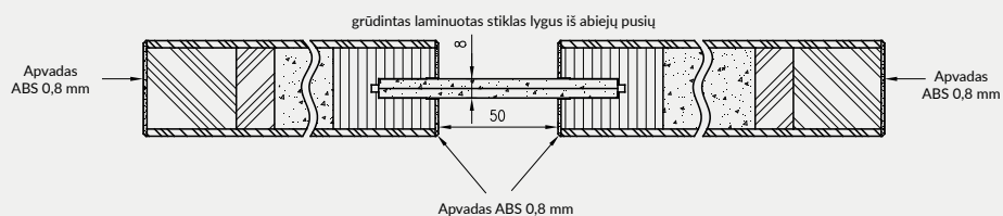
Horizontalus VETRO E duru pjūvis
