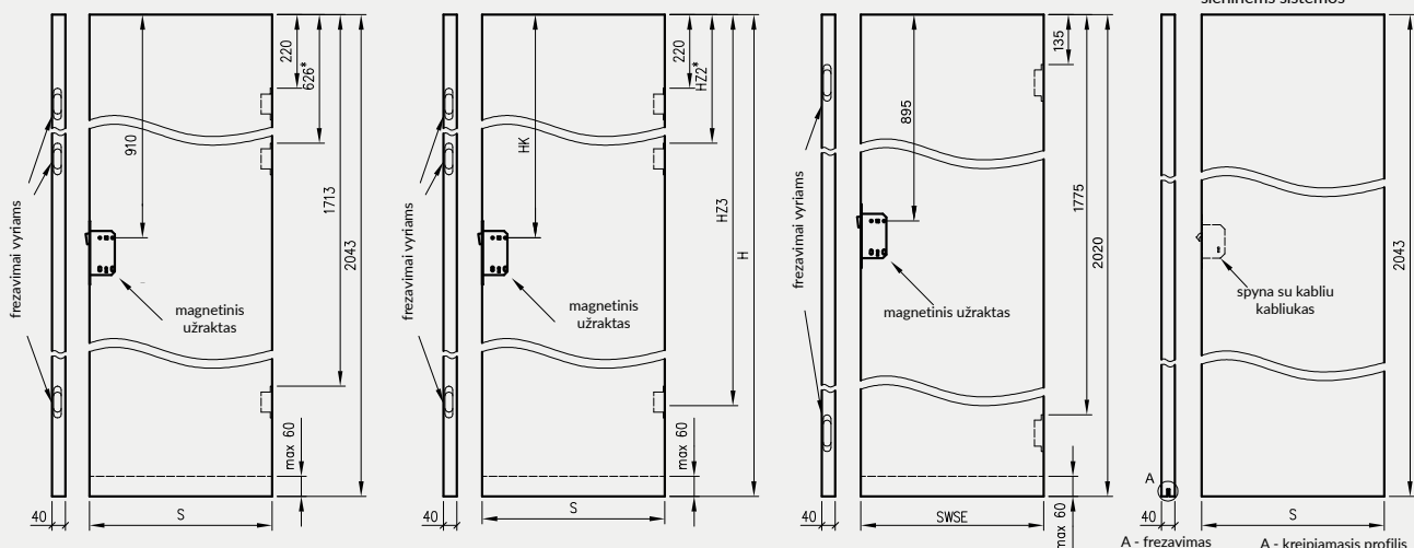
Atveriamos lygiabriaunės varčios Standard 10, Modern, Plus
