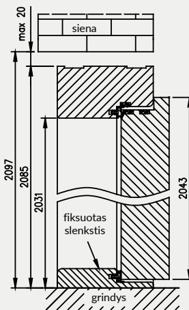
Medinė stakta „Athos“ durims su fiksuotu slenksčiu
