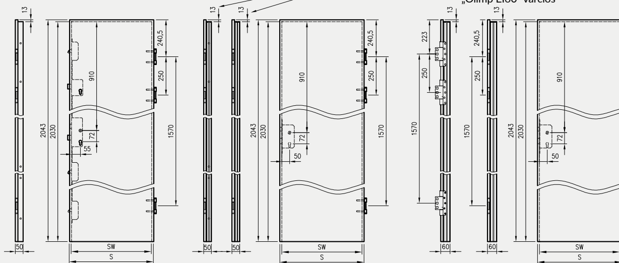
„Forca“ / „Forca B“ varčios
